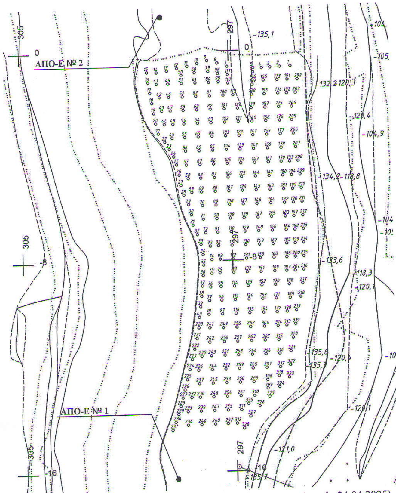
Рисунок 1 – Схема дослідного блоку (бл. № 21 гор. -150 м від 24.04.2025)
