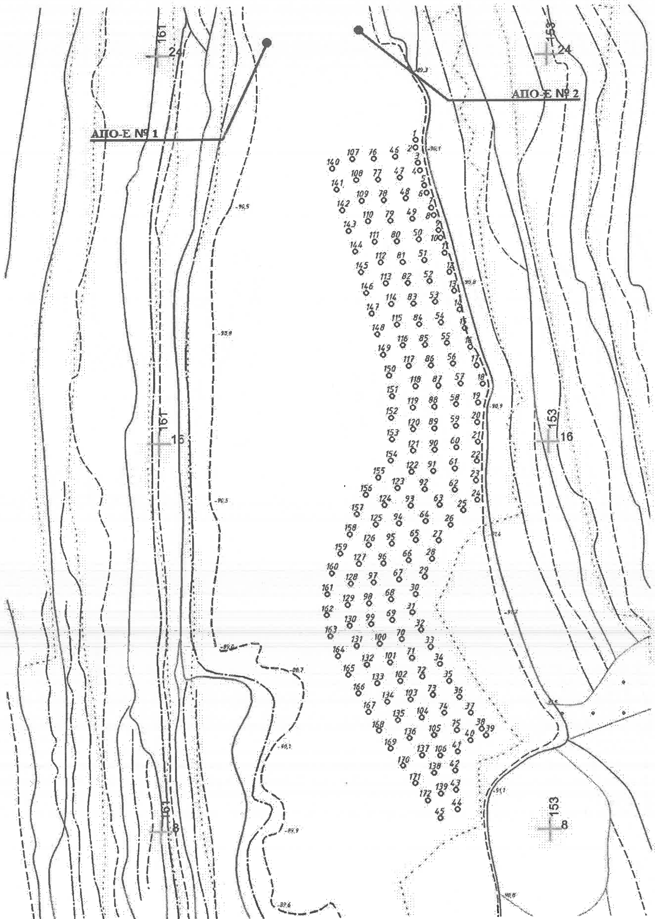
Рисунок 1 – Схема дослідного блоку (бл. № 6 гор. -105 м від 20.02.2025)
